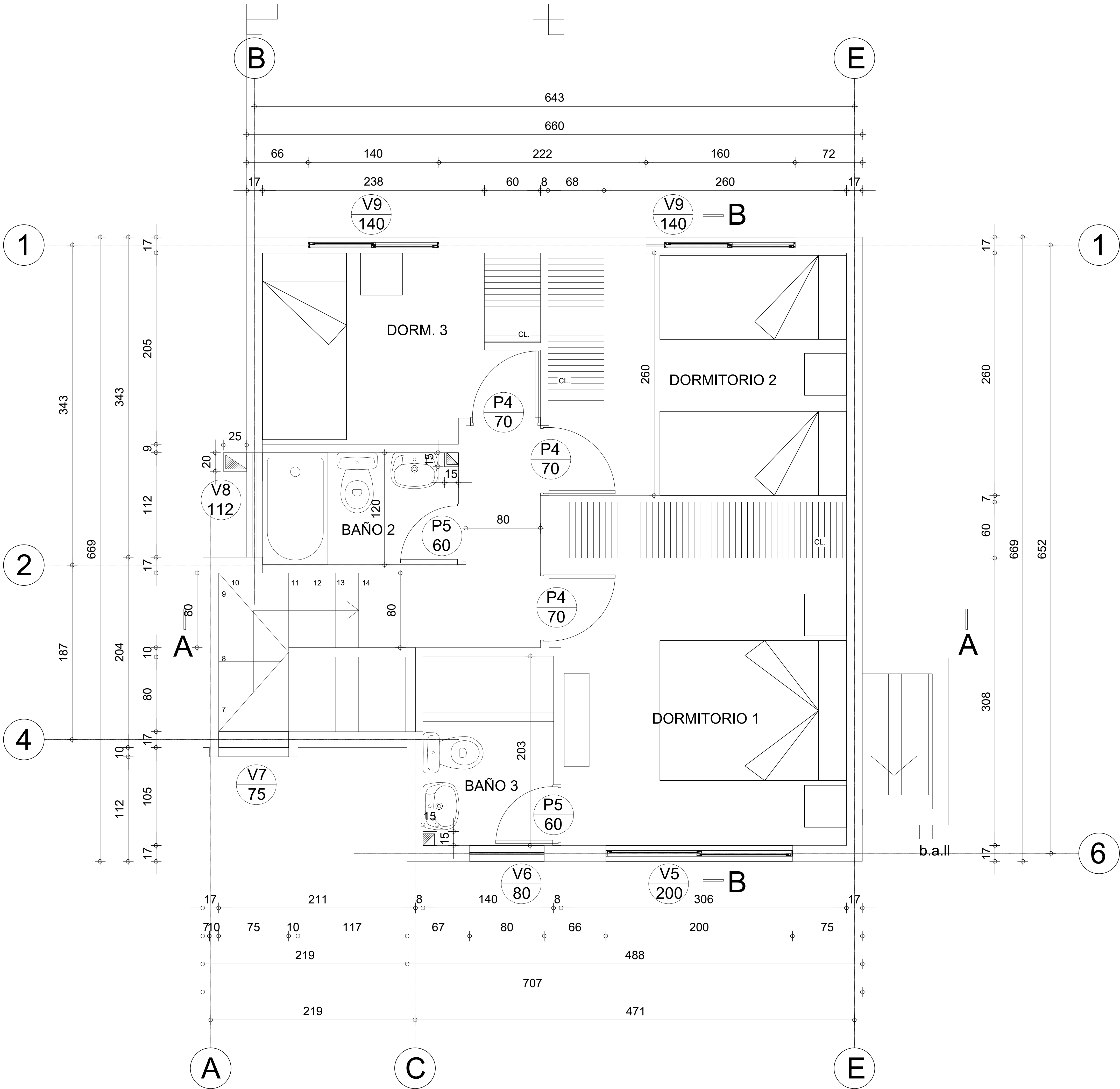
PLANTA SEGUNDO PISO ESCALA 1:50
